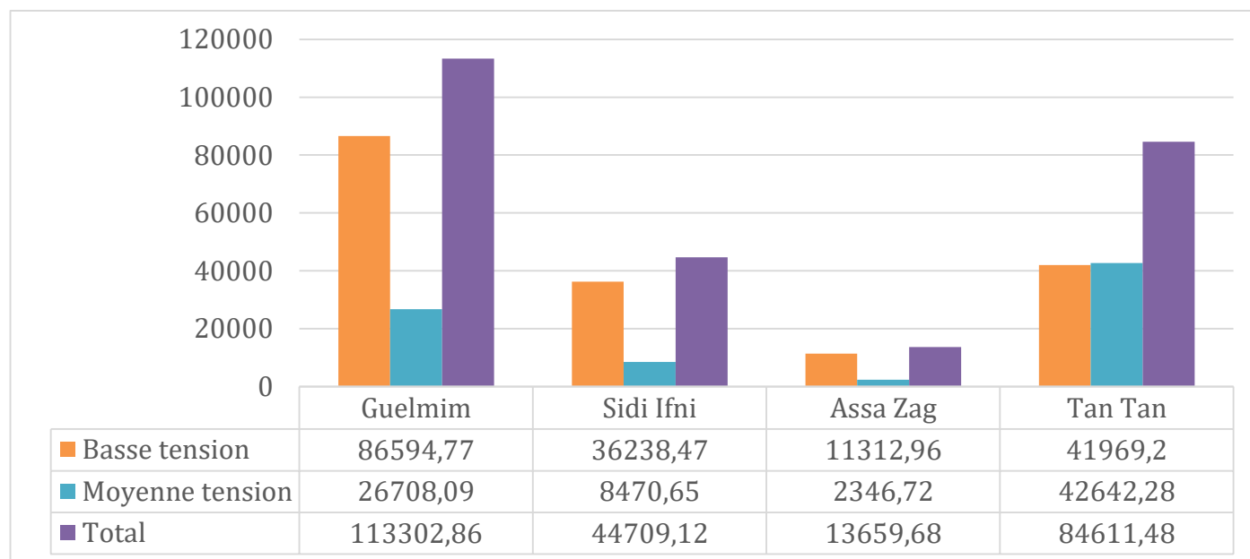
Figure 22: Vente totale d'énergie électrique (en MWH) en 2022
