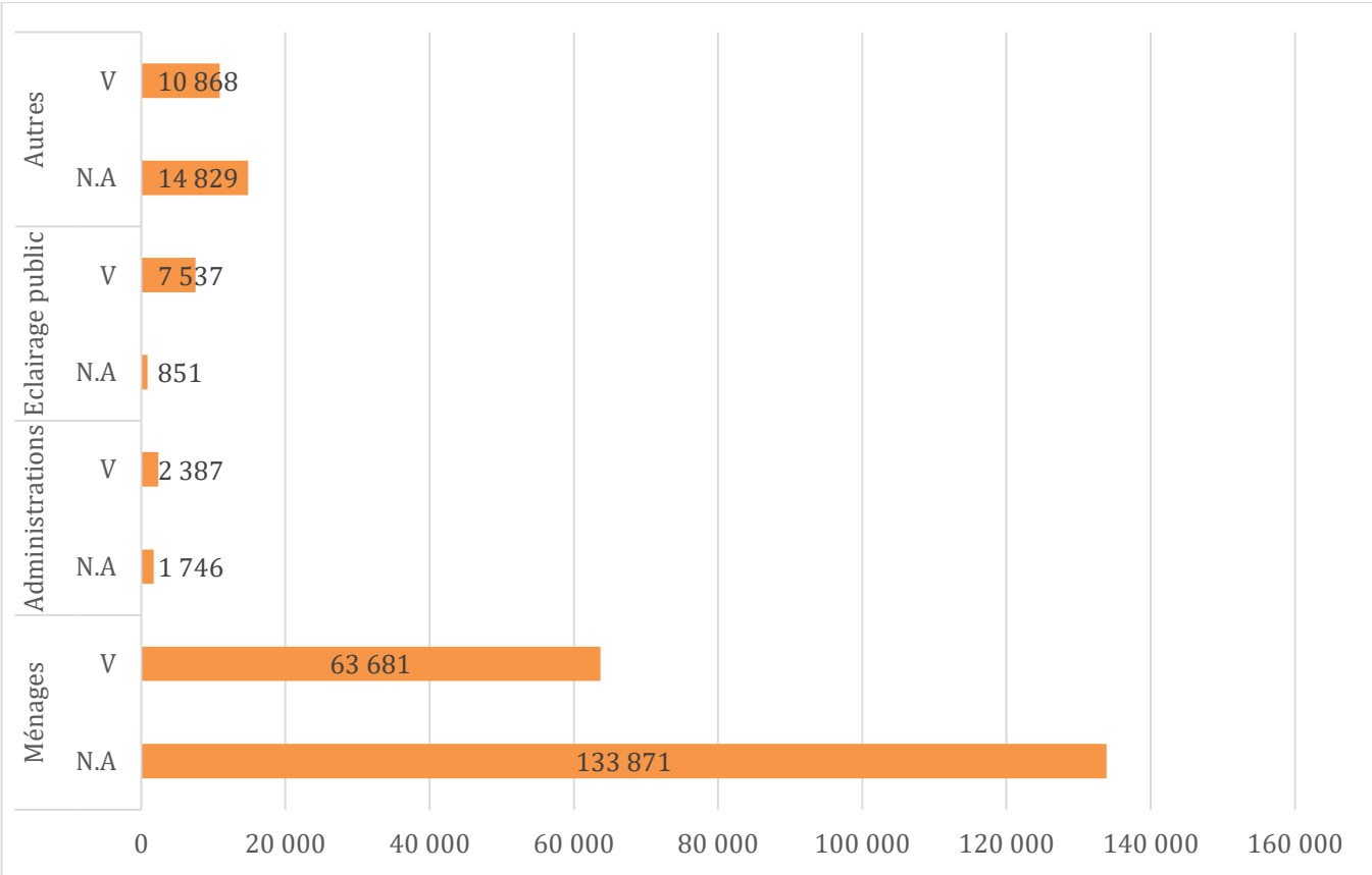
Figure 23: Structure de vente d'électricité (MWH) par groupes d'abonnés en 2022
